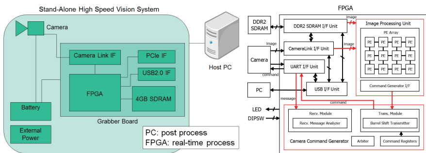
スタンドアロン高速ビジョンシステムおよびシステムに搭載されたFPGA内のブロック図 Block diagrams of Standalone High-Speed Vision System and FPGA on the system
