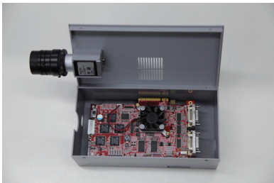
スタンドアロン高速ビジョンシステムの試作 Prototype of Standalone High-Speed Vision System
