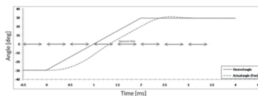
図2 応答時間測定実験の結果 Fig.2 Experimental Result
