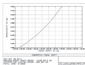
図 3 (左) 単一アダプティブレンズの色による焦点距離変動 Figure 3. (Left) Chromatic focal shift of Adaptive Singlet.
