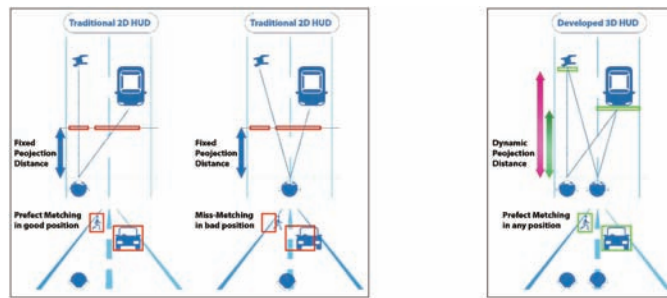
図1. (左図) 従来のHUDは、特定の注意情報をウインドウに映し出すことが可能だが、運転者の視線や速度に関係なく決まった奥行き位置に表示される。そのため運転手の視線がずれると、観測される表示にもずれが生じていた。(右図) 今回の技術では、高速投影技術を利用して三次元空間に虚像投影を行う。映像の表示位置を数 m ～数十 m などに変更可能であり、三次元的な空間表示となるためドライバーの視点位置が基準観察位置からずれても、AR 表示は情報を重畳させる対象からずれない。
